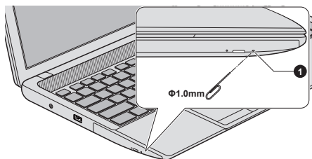
Рисунок 3-8 Открывание лотка вручную через отверстие для извлечения диска
