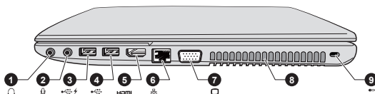
Рисунок 2-3 Правая сторона компьютера
