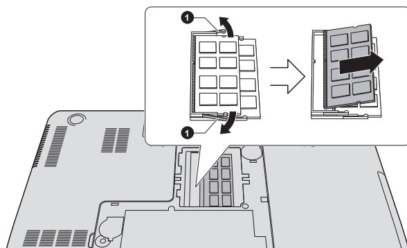
Рисунок 3-15 Удаление модуля памяти
