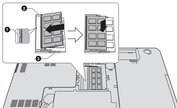
Рисунок 3-13 Установка модуля памяти
