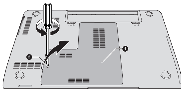
1. Крышка отсека модулей памяти 2. Винт
