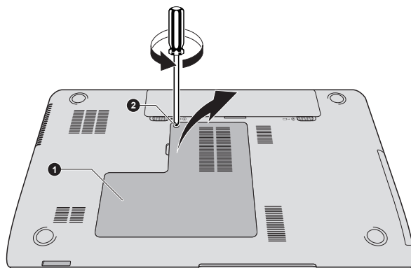
1. Крышка отсека модулей памяти 2. Винт
