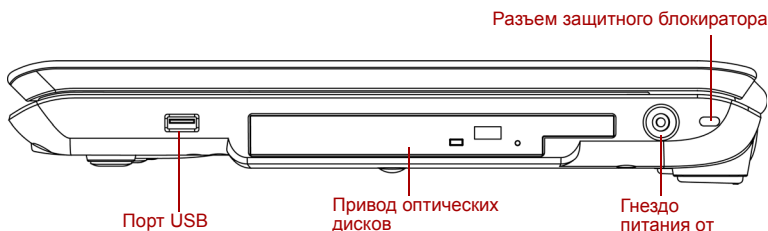
Рисунок 2-3 Вид компьютера справа
