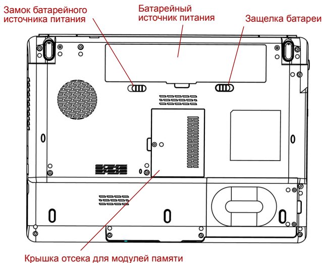
Рисунок 2-5 Вид компьютера снизу
