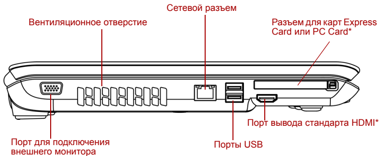
Рисунок 2-2 Вид компьютера слева
