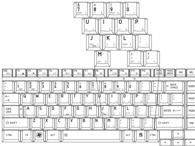
Рисунок 5-1 Цифровой сегмент клавиатуры
