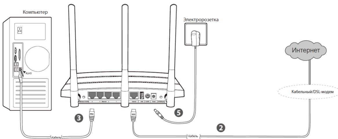
Рисунок 2-1 Установка аппаратной части маршрутизатора
