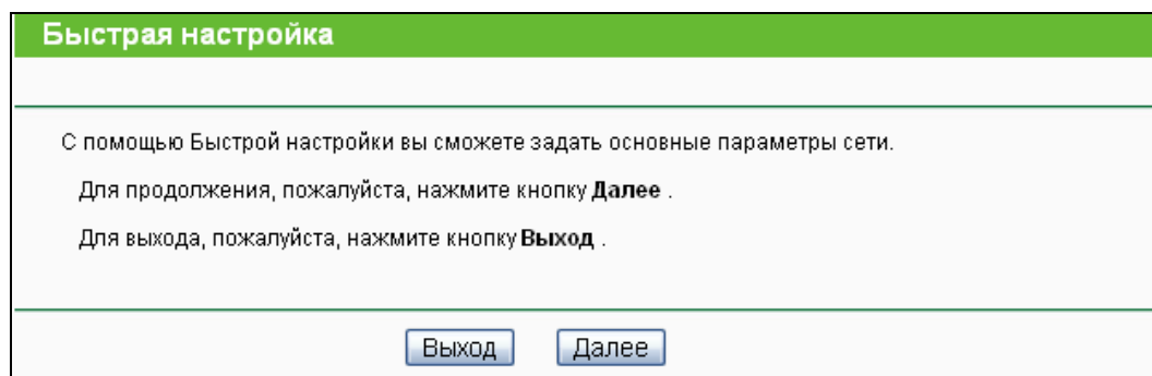
Рис. 3-5 Быстрая настройка
