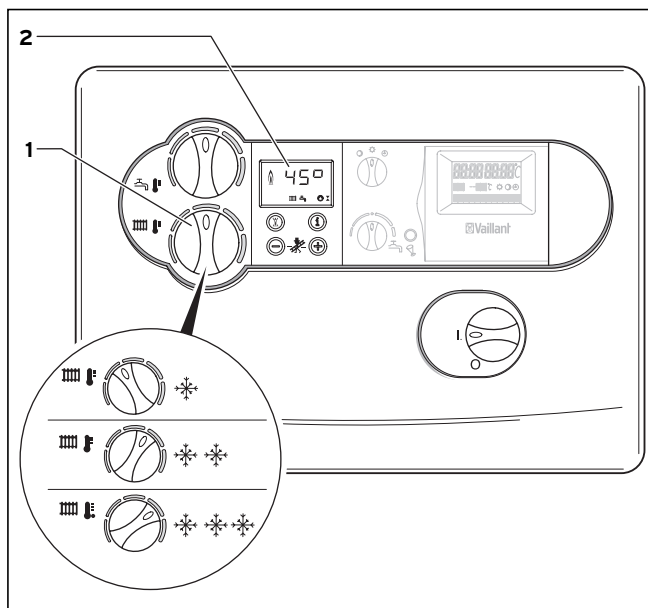
4.8 pav. Iš katilo ištekančio vandens temperatūros reguliavimas be reguliavimo prietaiso
