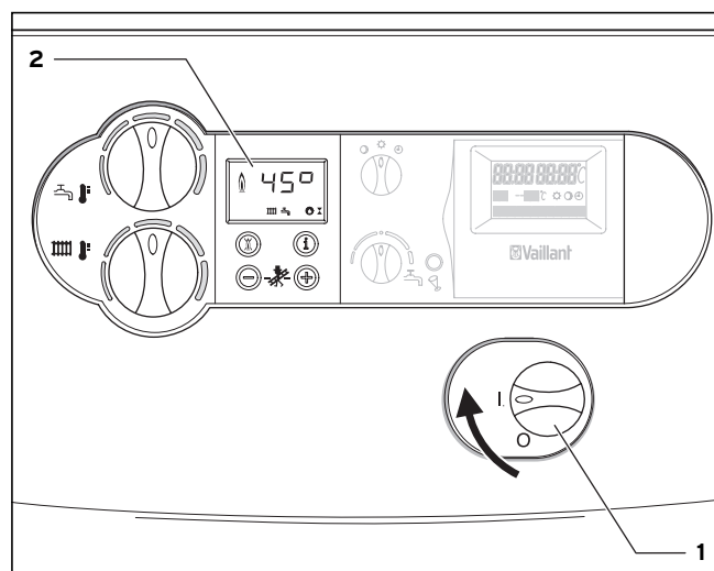
Рис. 4.5 Включение устройства
