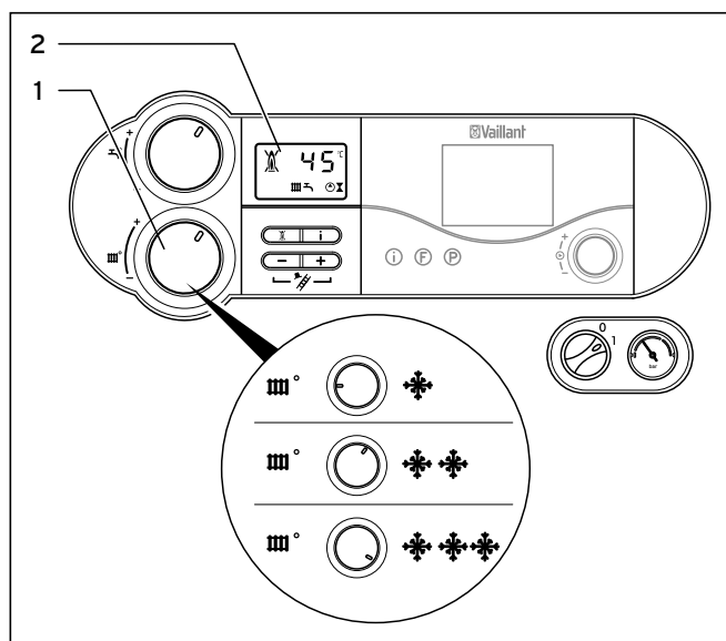
4.10 Настройка температуры теплоносителя в подающей линии без регулятора (показан аппарат atmoTEC/turboTEC plus)
