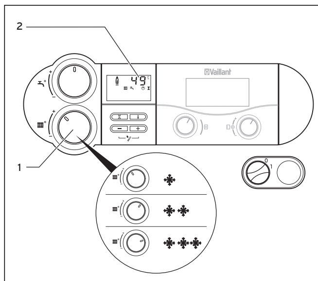
Мал. 4.8 Настроювання температури лінії подачі без регулювального пристрою
