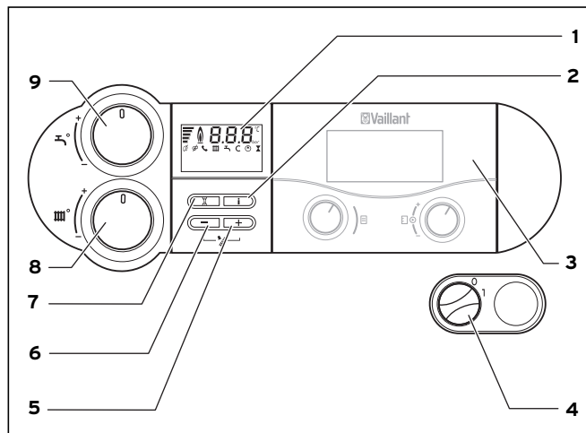
Fig. 4.1 Betjeningselementer på ecoVIT eksklusiv (eksempel)
