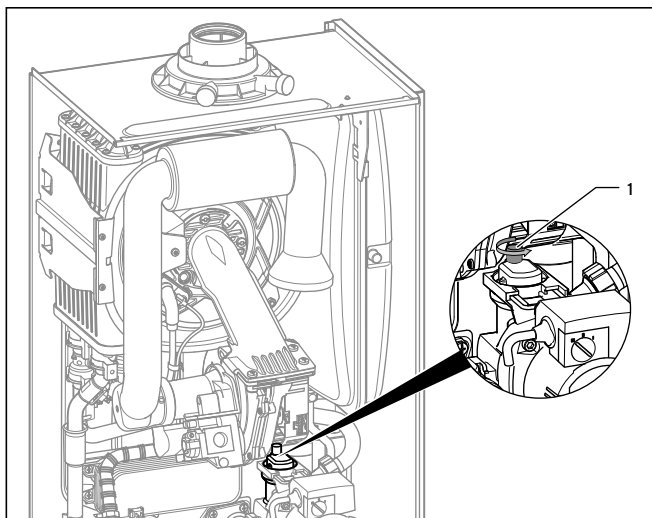
Рис. 6.2 Быстродействующий воздухоотводчик
