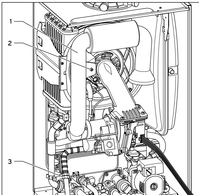
Рис. 8.1 Демонтаж воздуховсасывающей трубы
