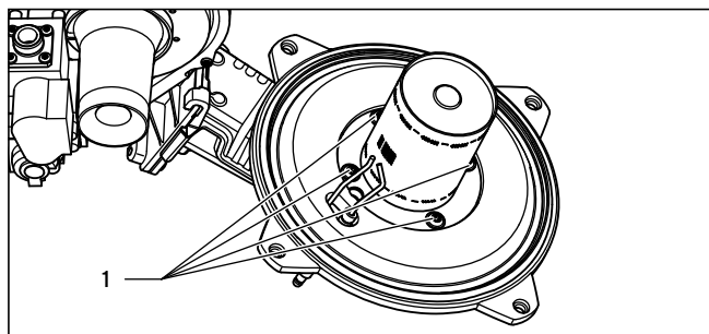
Рис. 10.1 Замена горелки
