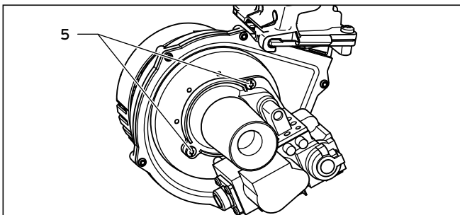
Рис. 10.3 Резьбовое соединение газовой арматуры/воздушная заслонка
