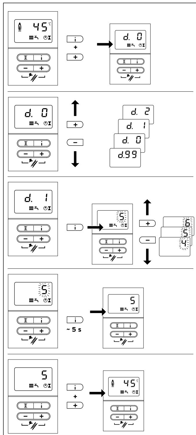
Рис. 7.1 Настройка параметров
