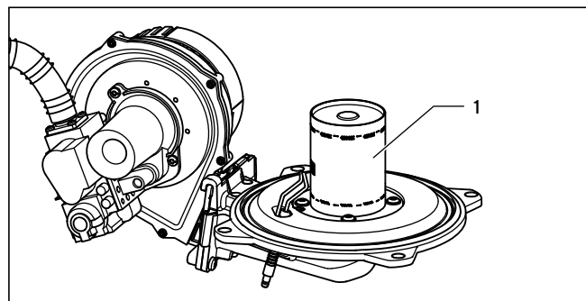
Рис. 8.4 Проверка горелки
