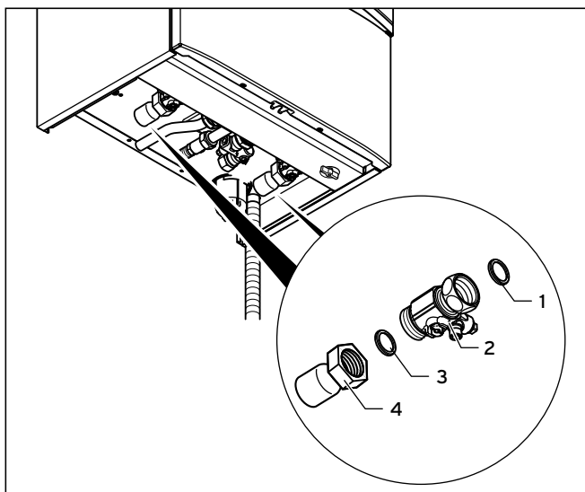
Рис. 5.4 Монтаж подающей и отводящей линий отопления (пример аппарат VUV)
