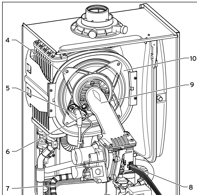
Рис. 8.2 Демонтаж компактного термомодуля
