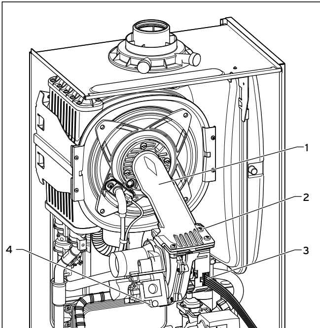
Рис. 10.2 Демонтаж воздушной заслонки с газовой арматурой
