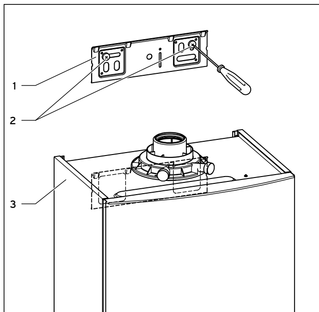
Рис. 4.6 Навешивание аппарата
