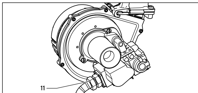
Рис. 8.8 Проверка газонепроницаемости
