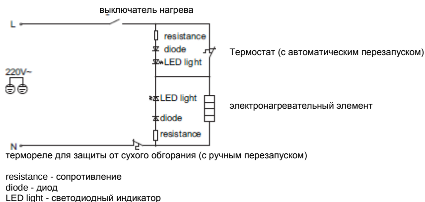
D26WF - Принципиальная электрическая схема
