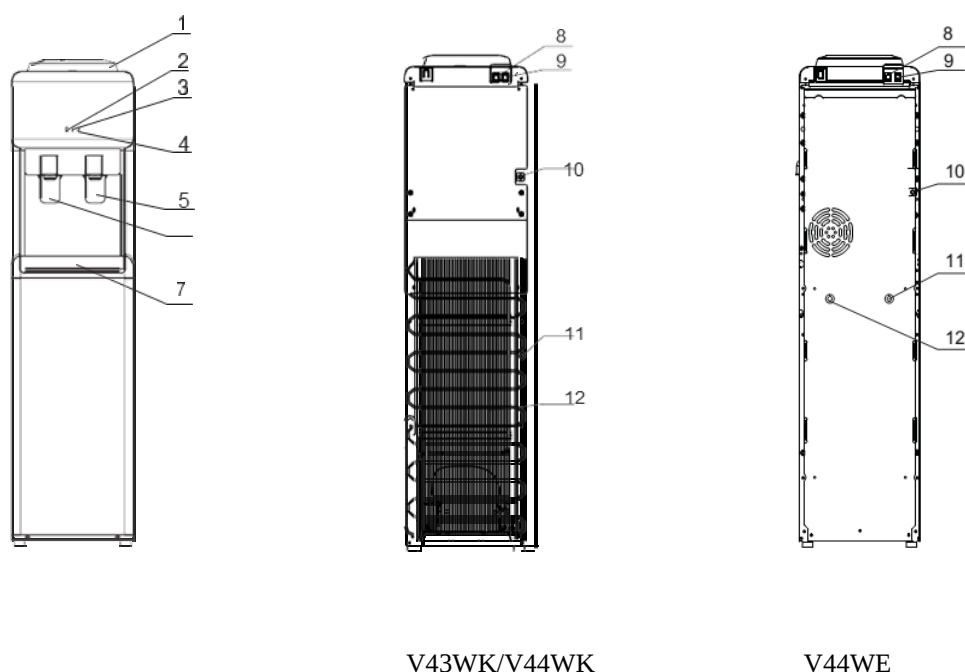
Рис.1 Наименование компонентов диспенсера V43WK/V44WK/V44WE
