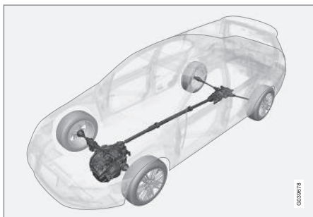
Принцип AWD - привод на все четыре колеса 10 .
