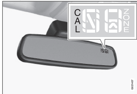
Калибровка компаса.
