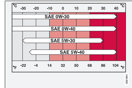
Диаграмма вязкости
