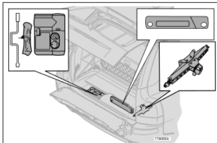
Пятиместная модель, на рисунке приведен вариант 1 шиноремонтного комплекта
