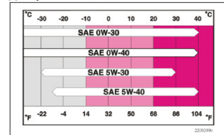
Диаграмма вязкости
