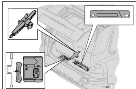
Семиместная модель, на рисунке приведен вариант 1 шиноремонтного комплекта
