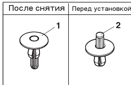
1. Пистон быстрого крепления 2. Штифт
