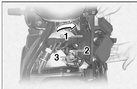
1. Панель блока зажигания 2. Запасной главный предохранитель 3. Главный предохранитель
