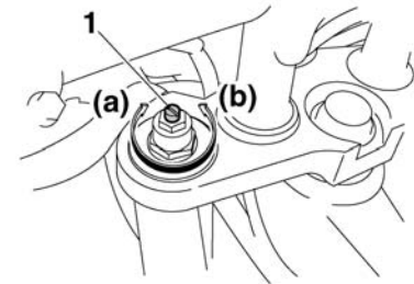
1. Винт регулировки хода сжатия
