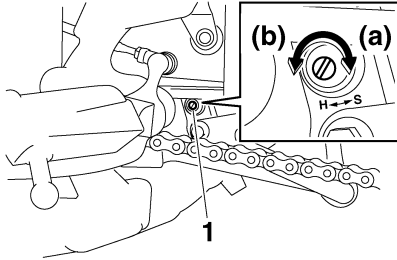
1. Винт регулировки хода отбоя
