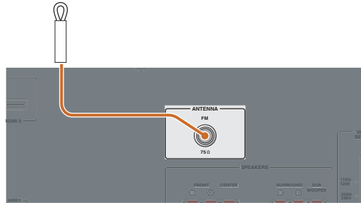
Комнатная FM-антенна
