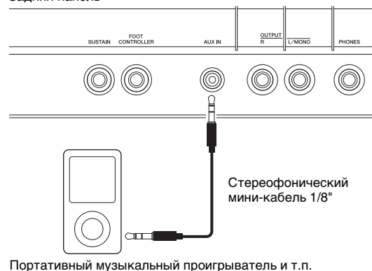
Задняя панель
