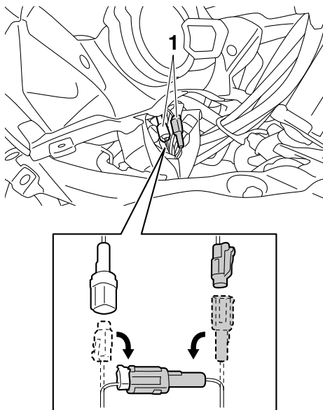
1. Разъем выключателя дроссельной заслонки
