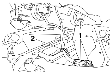
1. Электрический разъем фар 2. Пластмассовый пояс
