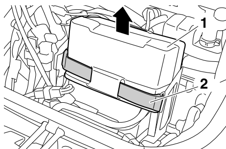
1. Крышка батарейного отсека 2. Лента крепления батареи
