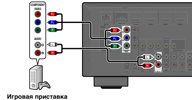
Компонентный видео-/аудиовыход
