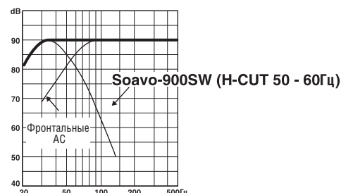
График частотной характеристики*
