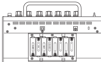
THR5/5A (Задняя сторона)
