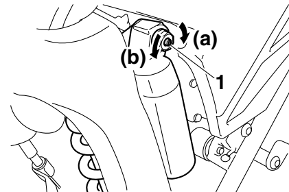
1. Регулировочный винт демпфирующей силы сжатия
