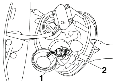
1. Разъём фары
