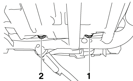
1. Болт слива масла А (картер): 2. Болт слива масла В (картер):
