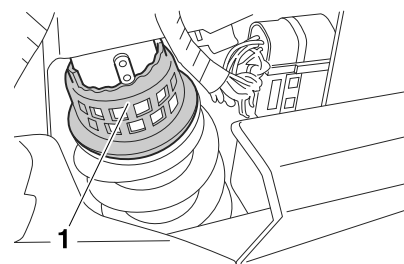
1. Регулировочное кольцо предварительной нагрузки пружины
