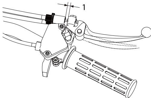
1. Свободный ход рычага переднего тормоза
