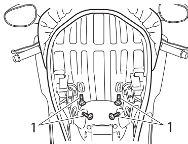
1. Болт
