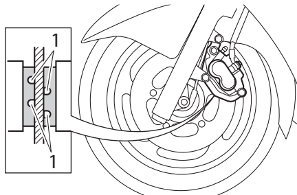
1. Индикатор износа
