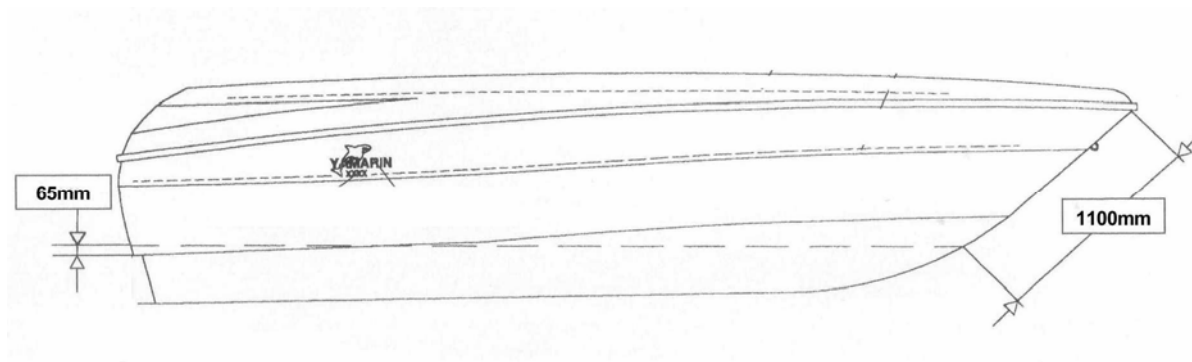
Ватерлиния судна Yamarin 53 Bow Rider
