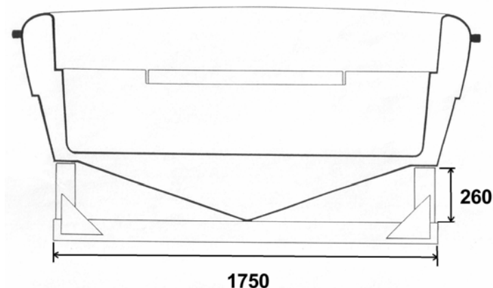
Размеры киль-блоков для судна YAMARIN 53 Bow Rider
