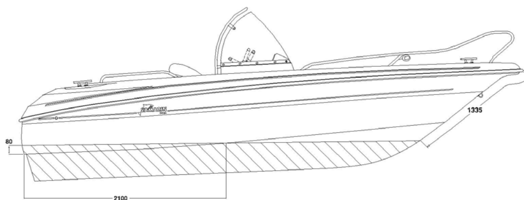
Ватерлиния
