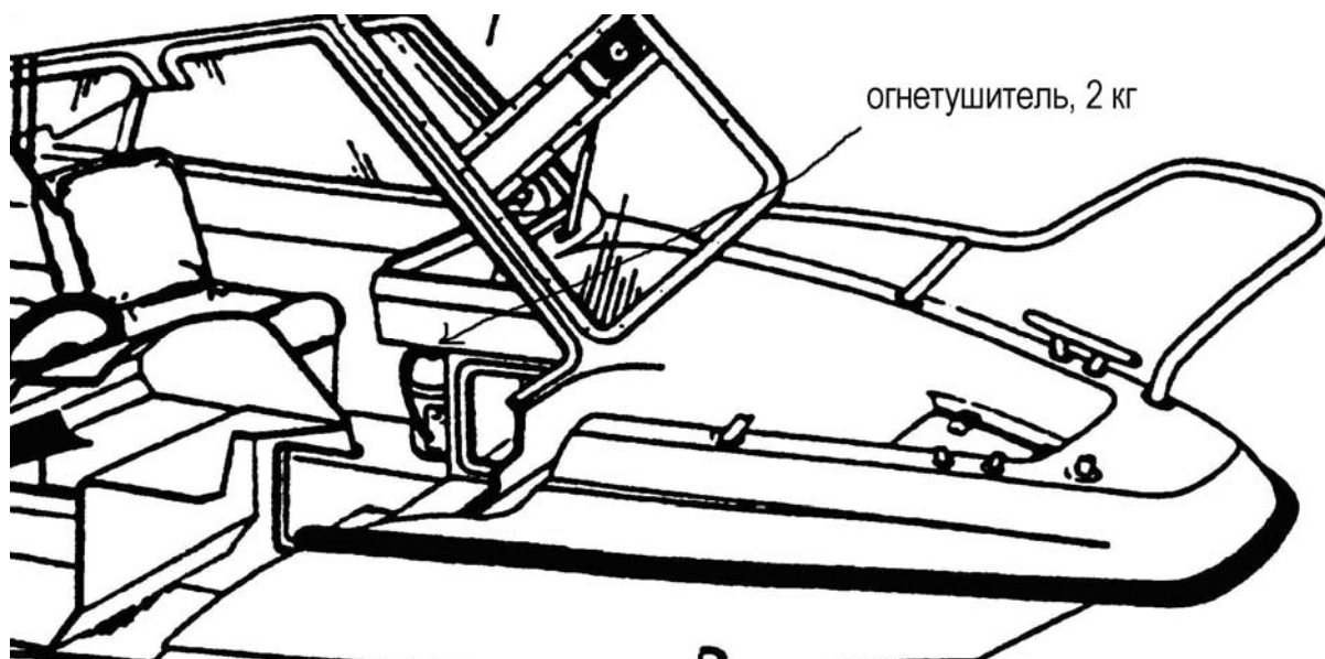
Расположение и объем огнетушителя на судне Yamarin 59 Cabin
