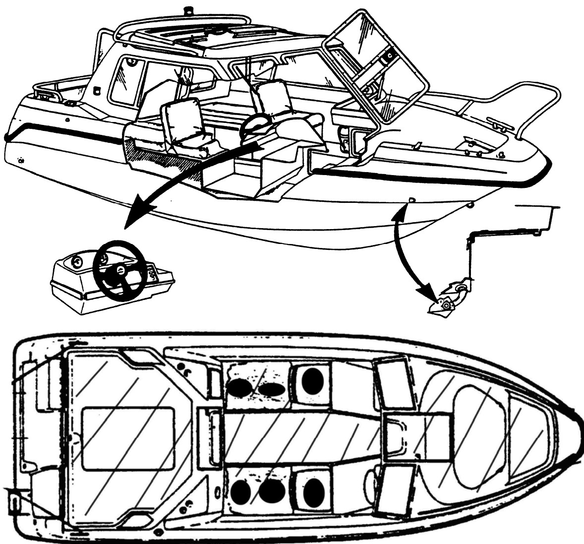
Основная палуба и рекомендуемое размещение людей на борту судна Yamarin 59 Cabin
