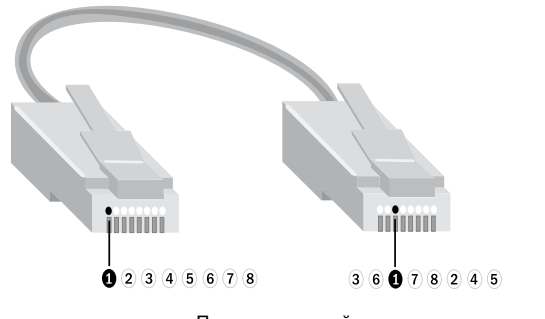
Перекрещенный кабель Ethernet
