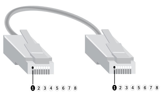
Прямой кабель Ethernet
