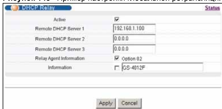
Рисунок 148 Пример настройки глобальной ретрансляции DHCP
