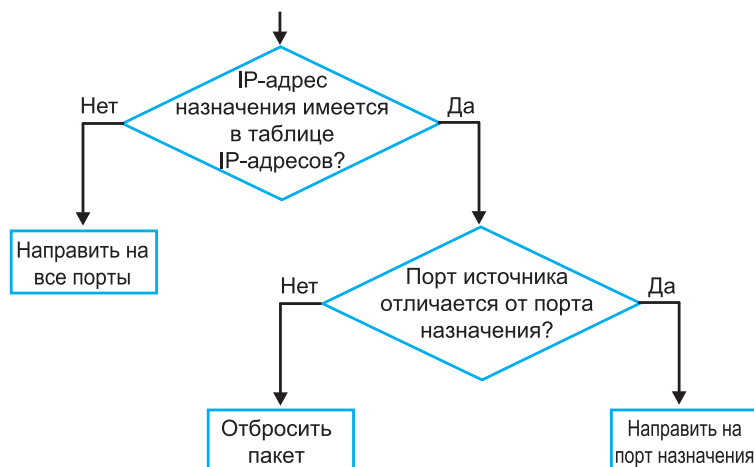
Рисунок 197 Схема работы таблицы IP-адресов
