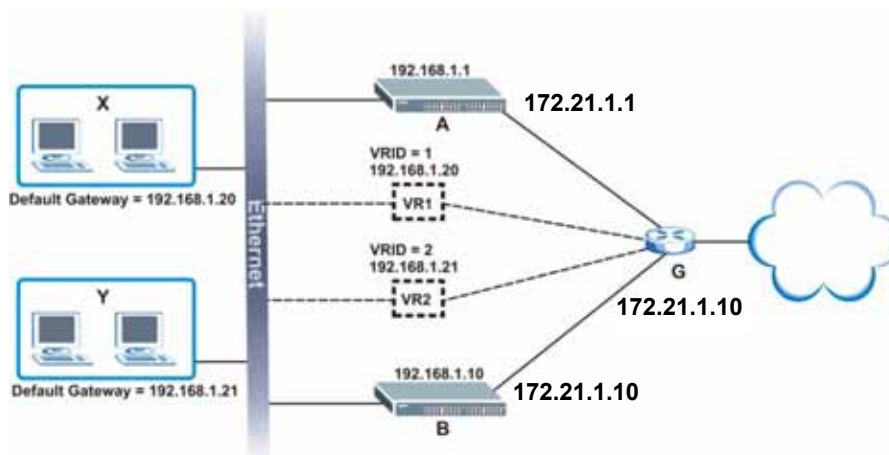
Рисунок 162 Пример настройки VRRP: сеть с двумя виртуальными маршрутизаторами
