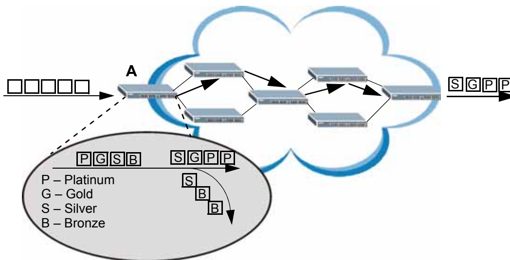
Рисунок 138 Сеть с поддержкой DiffServ
