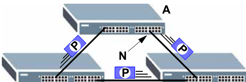
Рисунок 115 Защита от образования петель – петля в сети
