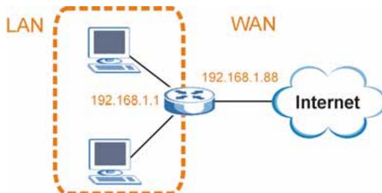
Рисунок 215 Пример с конфликтом IP-адресов маршрутизатора
