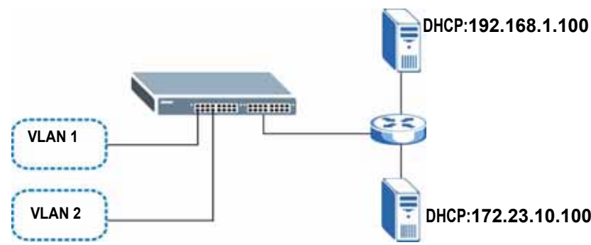
Рисунок 150 Ретрансляция DHCP для двух VLAN
