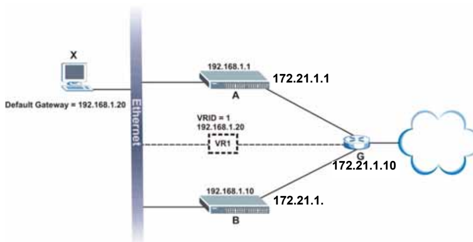
Рисунок 157 Пример настройки VRRP: сеть с одним виртуальным маршрутизатором
