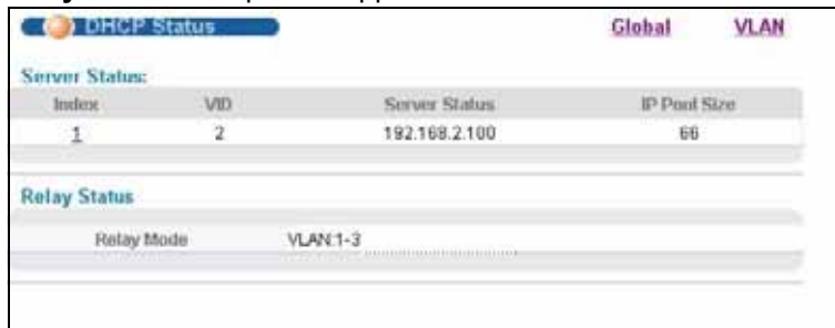
Рисунок 144 Экран IP Application > DHCP Status
