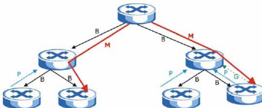
Рисунок 131 Как работает протокол DVMRP
