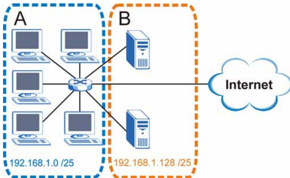
Рисунок 213 Пример формирования подсетей: после деления на подсети
