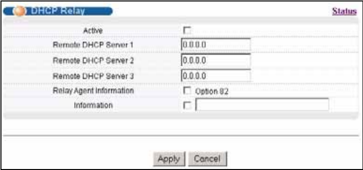
Рисунок 146 Экран IP Application > DHCP > Global
