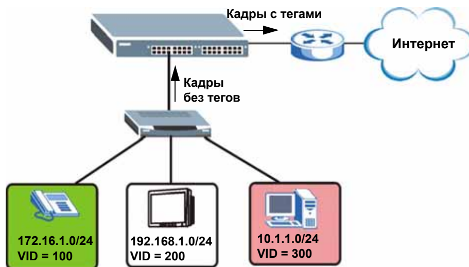
Рисунок 39 Пример использования VLAN на основе подсетей
