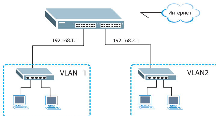
Рисунок 23 Пример первичной настройки сети: IP-интерфейс
