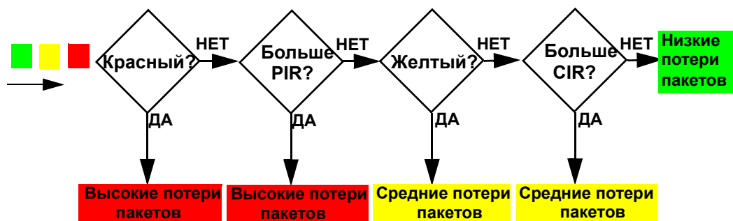
Рисунок 140 TRTCM – режим с учетом цвета
