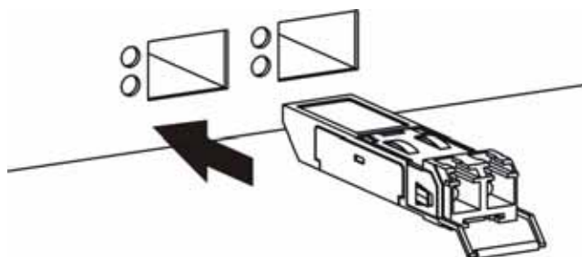
Рисунок 10 Пример установки трансивера
