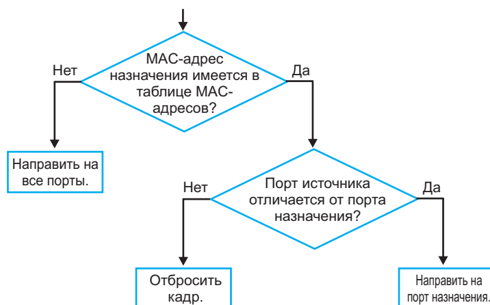
Рисунок 195 Схема работы таблицы MAC-адресов
