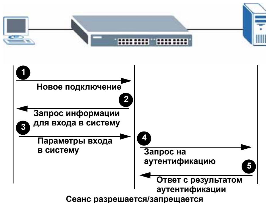
Рисунок 66 Процесс аутентификации на основе IEEE 802.1x
