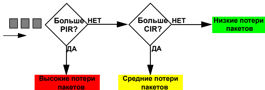
Рисунок 139 TRTCM – режим без учета цвета
