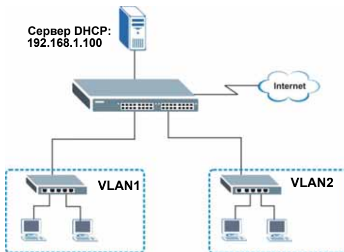
Рисунок 147 Пример сети с глобальной ретрансляцией DHCP
