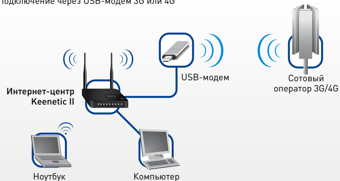
Подключение через USB-модем 3G или 4G
