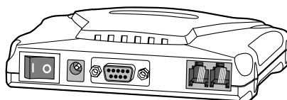
Задняя панель модема Omni 56K Neo
