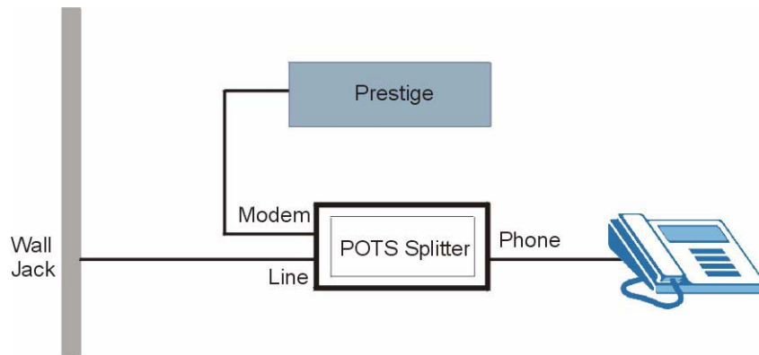
Рис. 5 Сплиттер
