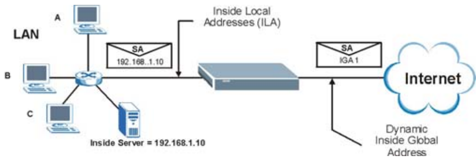
Рис. 30-13 Пример 2 NAT
