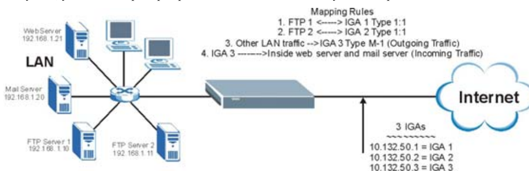
Рис. 30-15 Пример 3 NAT
