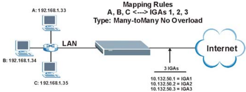
Рис. 30-19 Пример 4 NAT
