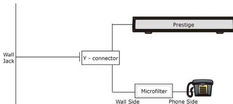
Схема 49-2 Подключение микрофильтра
