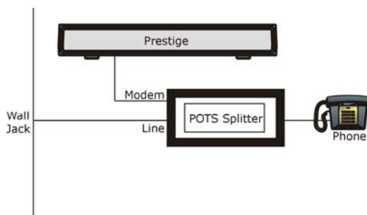
Схема 49-1 Подключение разделителя частот POTS
