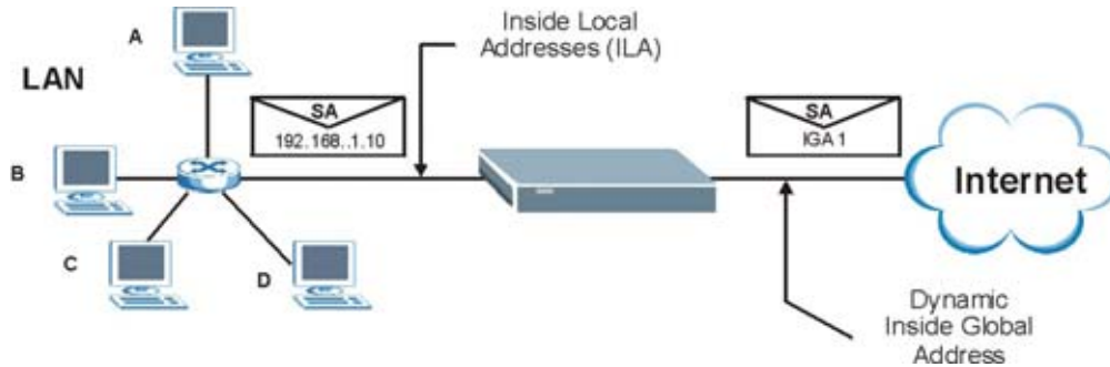
Рис. 30-11 Пример 1 NAT
