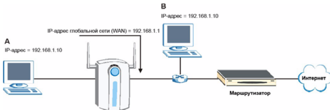
Рис. 231 Конфликты IP-адресов: случай С
