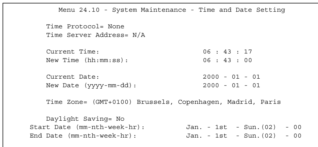
Рис. 183 Меню 24.10: управление системой – настройка времени и даты
