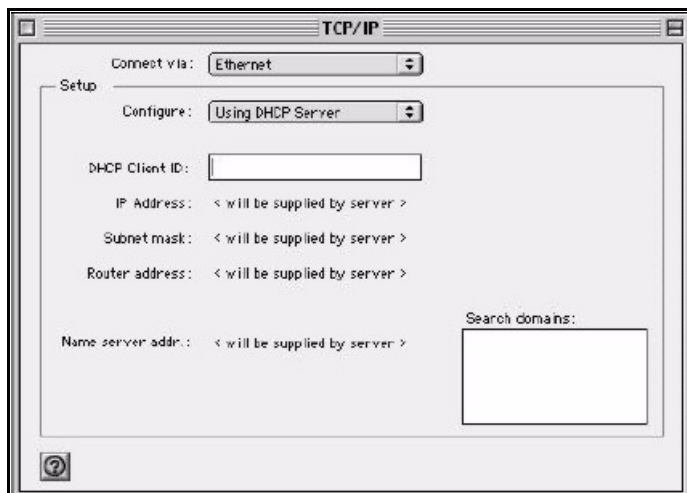
Рис. 206 Macintosh OS 8/9: TCP/IP
