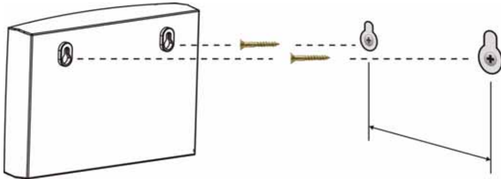
Рис. 193 Пример монтажа на стене
