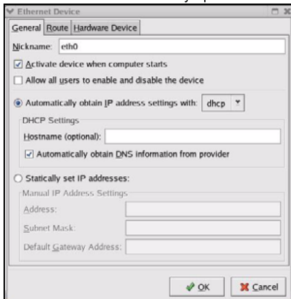
Рис. 210 Red Hat 9.0: KDE: устройство Ethernet: общие настройки
