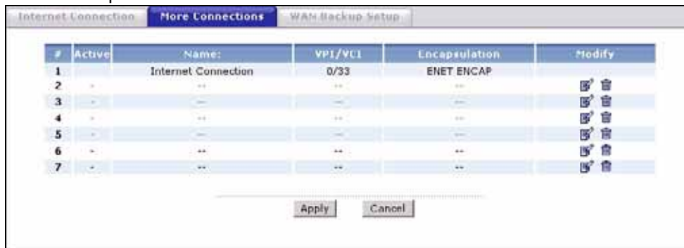
Рис. 25 Экран WAN > More Connections
