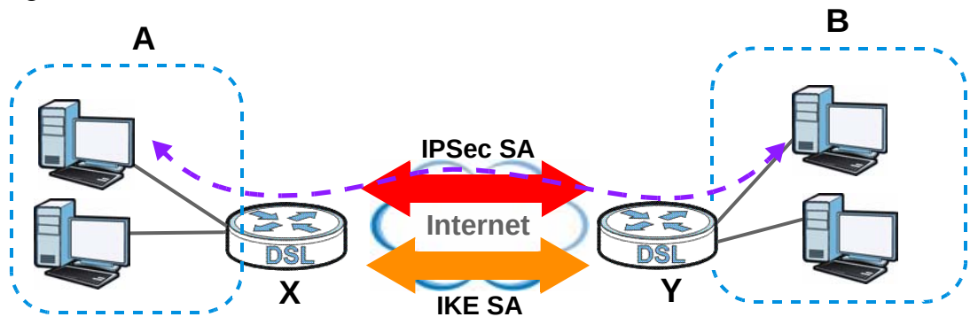
Figure 70 VPN: IKE SA and IPSec SA
